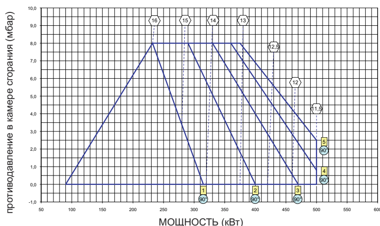
ПРИМЕР ПРЕДВАРИТЕЛЬНОЙ КАЛИБРОВКИ MAX GAS 500 PAB
