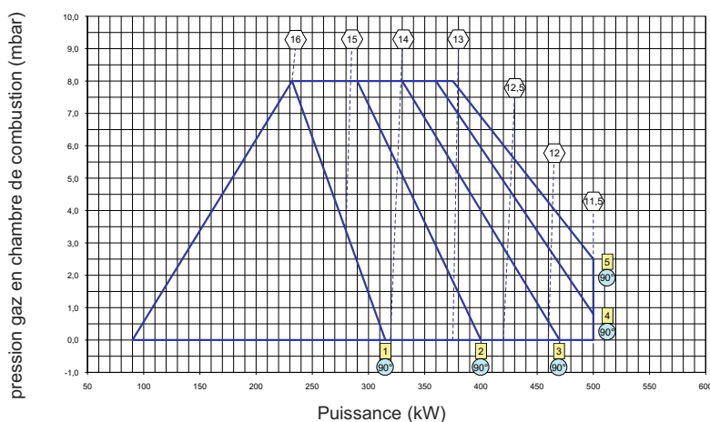
EXEMPLE DE PREREGLAGE MAX GAS 500 PAB
